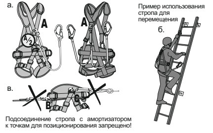
Рис. 5. Использование стропа с амортизатором рывка
