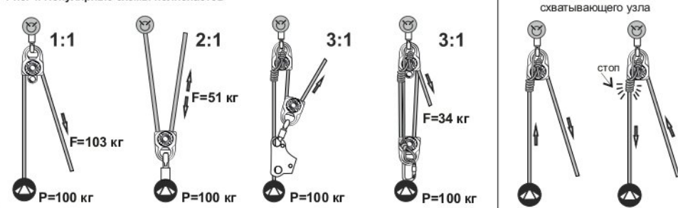
Рис. 4. Популярные схемы полиспастов
