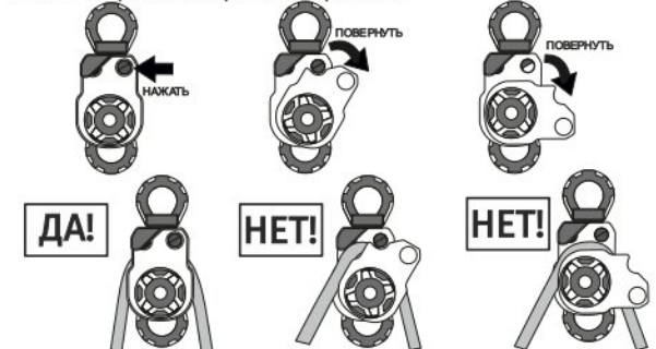
Рис. 6. Раскрытие блок-ролика с вертлюгом
