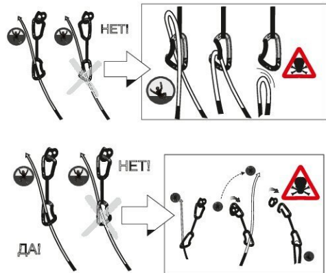
Рис. 3. Процеживание веревки
