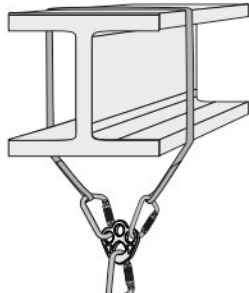
Рис. 3. Использование такелажной пластины
