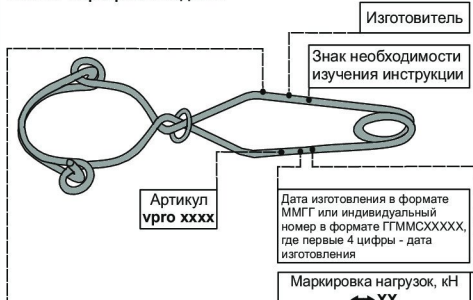
Рис. 2. Маркировка изделий
