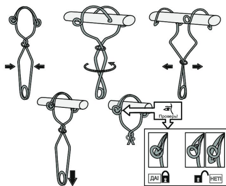
Рис. 3. Открытие / закрытие / фиксация запорного элемента трубного карабина
