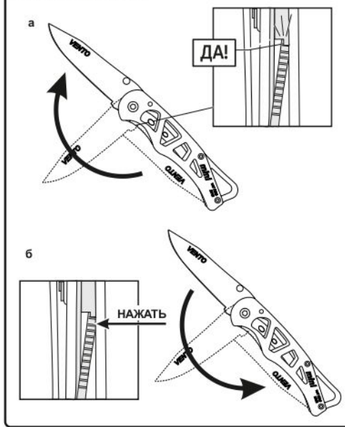
Рис. 2. Принцип работы
