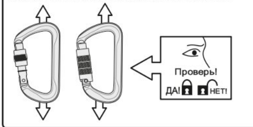
Рис. 5. Приложение нагрузки для карабинов класса В
