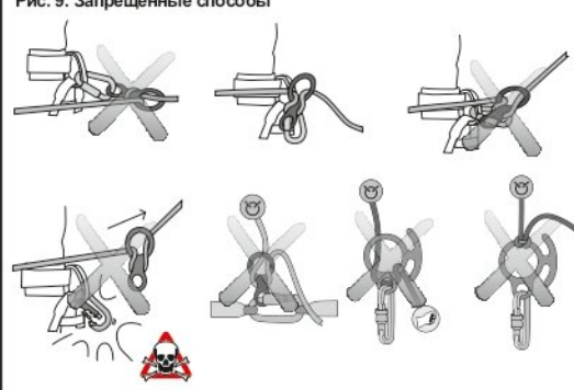
Рис. 9. Запрещенные способы
