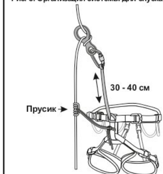
Рис. 8. Организация системы для спуска
