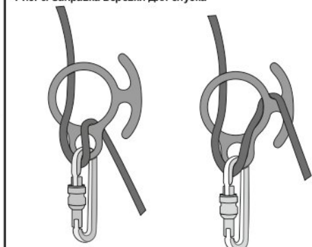
Рис. 6. Заправка веревки для спуска
