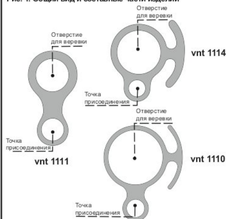
Рис. 2. Маркировка изделия
