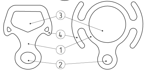
Рис. 1. 1 – тело спускового устройства; 2 – отверстие для присоединения карабина; 3 – отверстие для веревки; 4 – поверхности дополнительного торможения («рога»).
