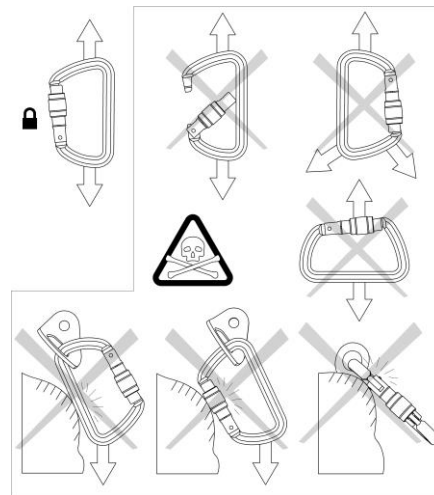
Рис. 7. Использование карабина
