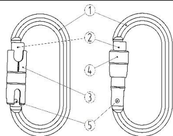
Рис. 1. 1 – скоба; 2 – защелка; 3 – автоматическая муфта; 4 – резьбовая муфта; 5 – ось.
