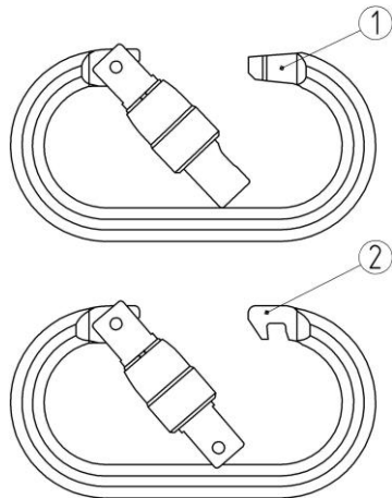
Рис. 2. Типы скоб. 1 – скоба keylock; 2 – скоба с крючком
