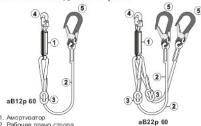
Рис. 1. Внешний вид, состав стропов
