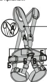
Рис. 3. Расположение и назначение крепежных точек на привязях
