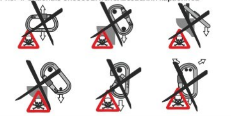
Рис. 4. Опасные способы использования карабинов
