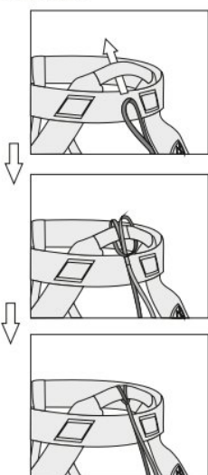
Рис. 3. Крепление усов
