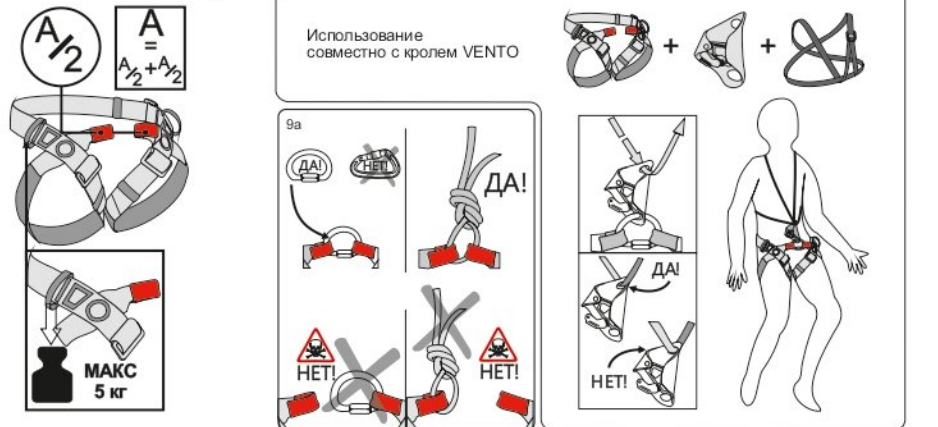
Рис. 7. Использование спелео-беседок
