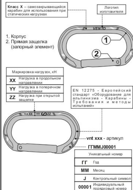
Рис. 1. Внешний вид, составные части, маркировка и характеристики карабина
