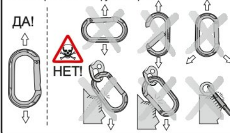
Рис. 2. Приложение нагрузки к карабинам
