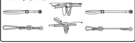
Рис. 10. Регулировка длины
