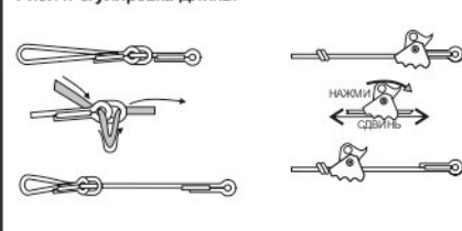
Рис. 7. Регулировка длины
