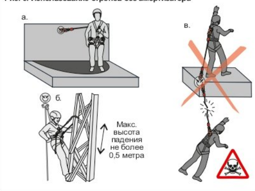
Рис. 9. Использование стропов без амортизатора
