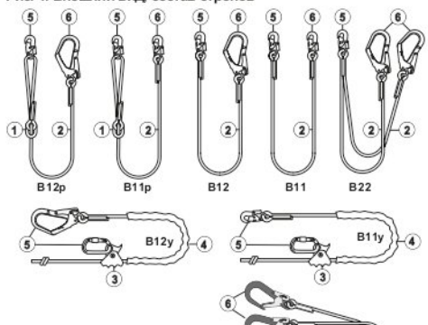
Рис. 1. Внешний вид, состав стропов
