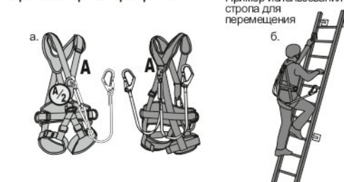
Рис. 4. В страховочных системах допускается использование только стропы с амортизатором рывка
