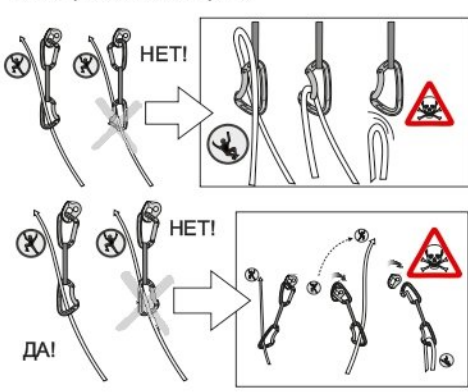
Рис. 7. Прощелкивание веревки
