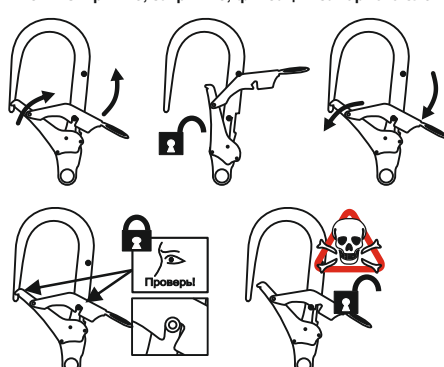
Рис. 2. Открытие, закрытие, фиксация запорного элемента
