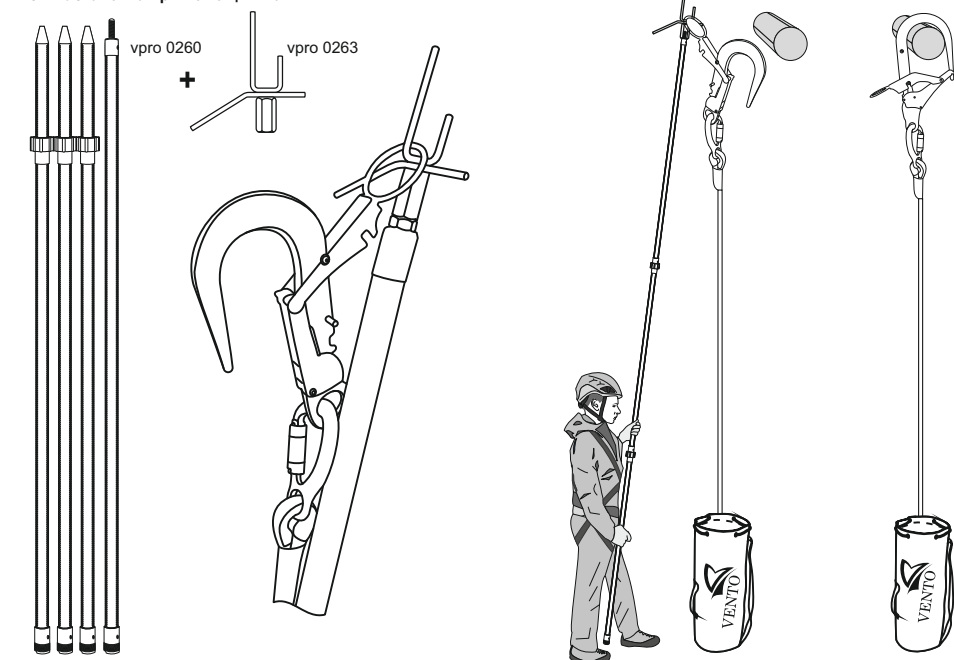
Рис. 4. Установка при помощи штанги
