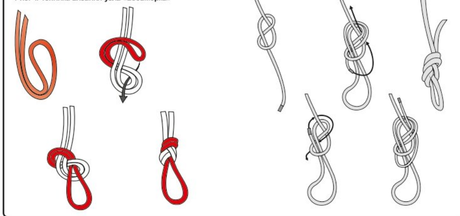
Рис. 4. Техника вязания узла «восьмерка»
