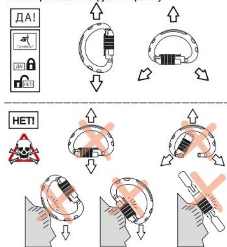
Рис. 3. Приложение нагрузки к карабину
