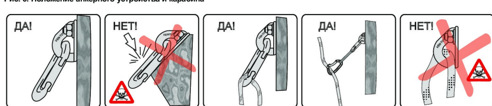
Рис. 6. Положение анкерного устройства и карабина
