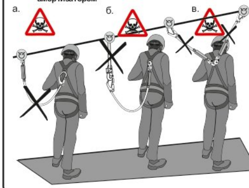
Рис. 10. Регулировка длины
