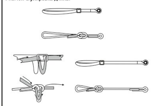
Рис. 10. Регулировка длины
