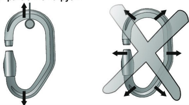
Рис. 4. Направление нагрузки
