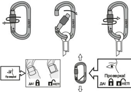
Рис. 3. Использование карабинов
