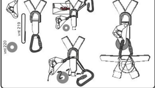
Рис. 11. Вариант интеграции зажима «Кроль» (требуется смена карабина угро 0224 с пилом на аналогичный без пина)
