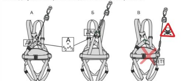
Рис. 4. Допустимые варианты соединения «НВ-02» с привязью
