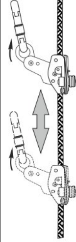
Рис. 6. Движение зажима вниз
