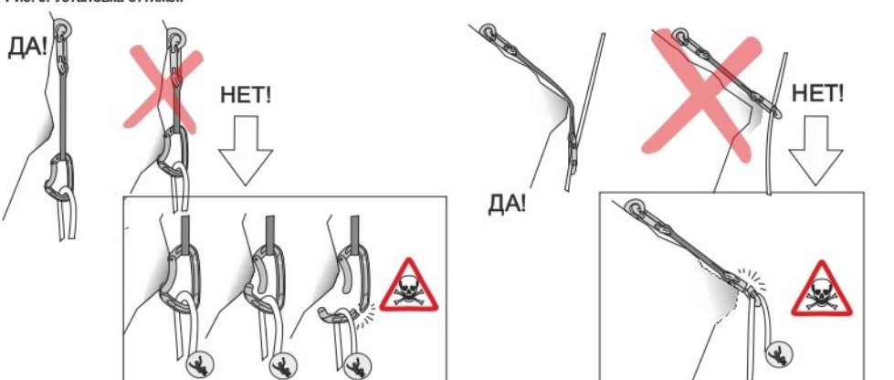
Рис. 6. Установка оттяжек
