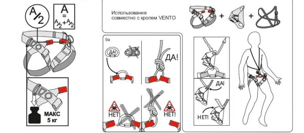
Рис. 7. Использование спелео-беседок
