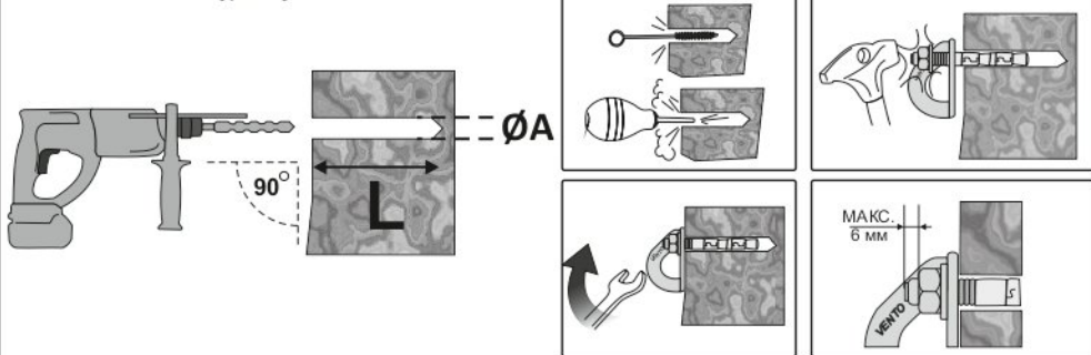
Рис. 3. Установка шлямбурного уха
