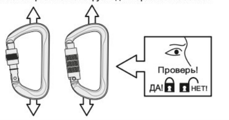
Рис. 5. Приложение нагрузки для карабинов класса В
