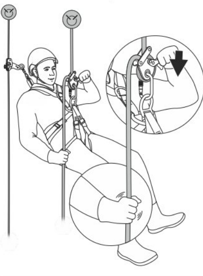
Рис. 10. Контроль каната
