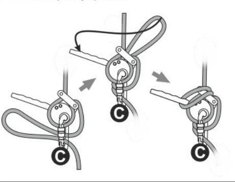
Рис. 13. Блокировка устройства
