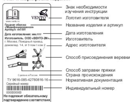
Рис. 1. Маркировка изделия
