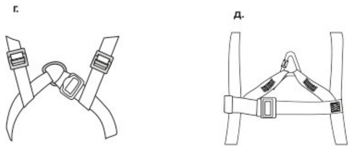
Рис. 11. Блокировка страховочной точки А на груди Альфа 1.5, 2.5, 1.5К, 2.5К
