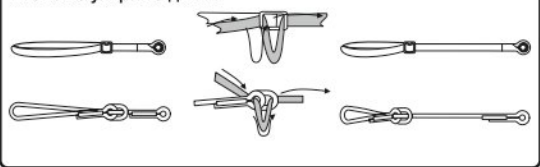
Рис. 10. Регулировка длины
