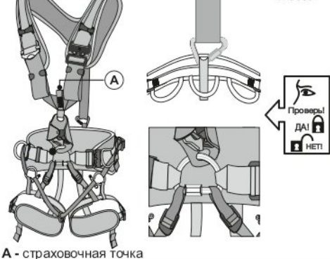
Рис. 2. Компоненты страховочной привязи «Профи Пихта» vnt 058
