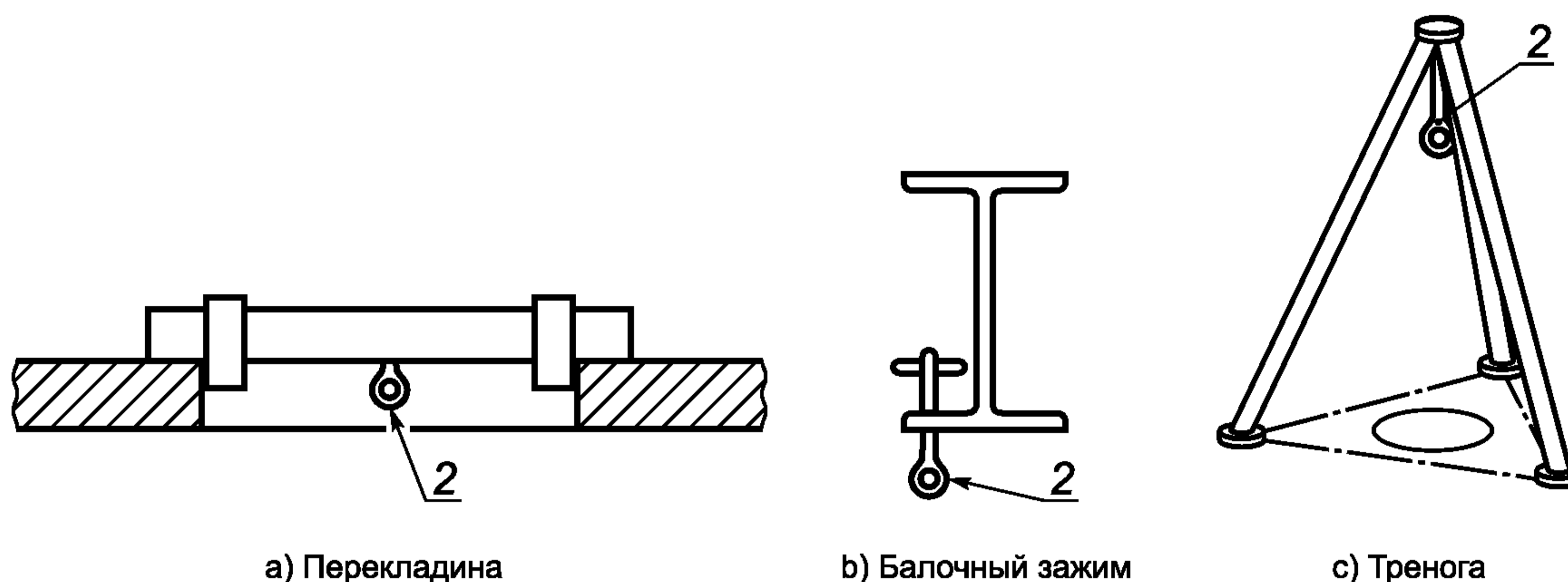
2 — точка анкерного крепления
