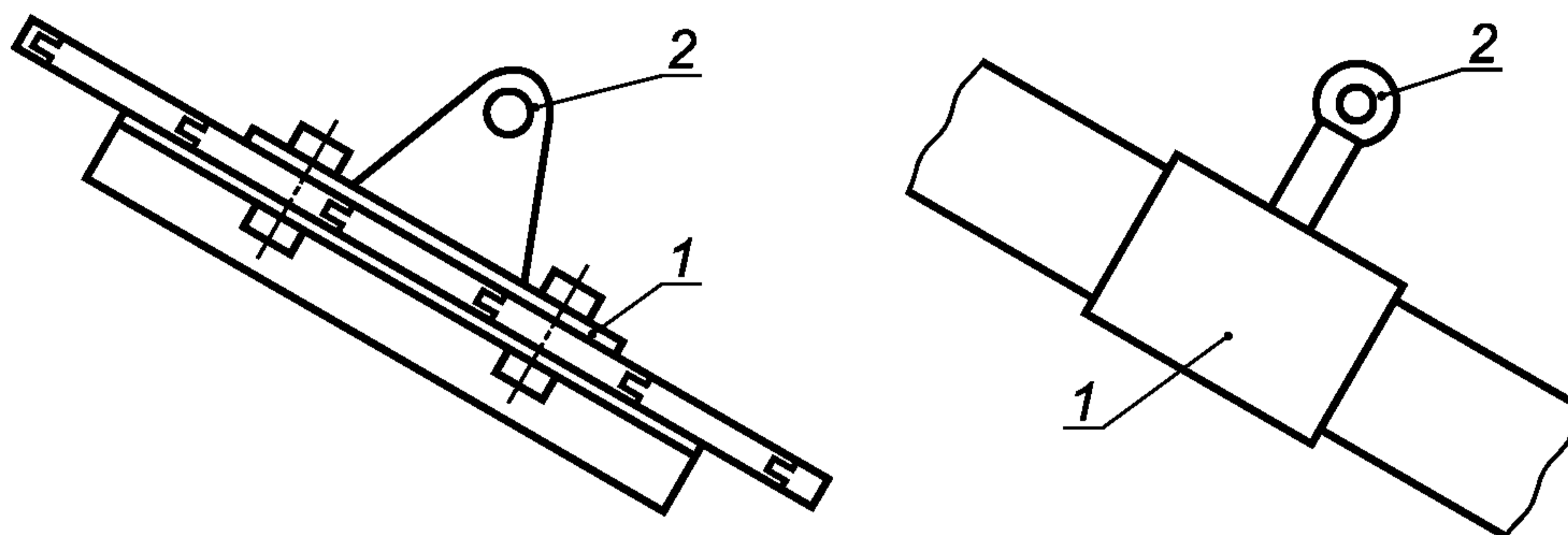
1 — структурный анкер; 2 — точка анкерного крепления
