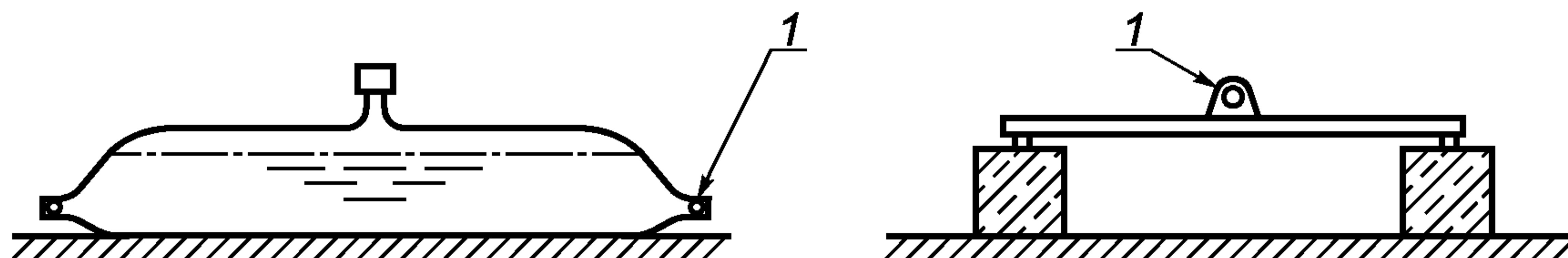
Рисунок 6 — Класс E. Примеры анкерных устройств с противовесом
