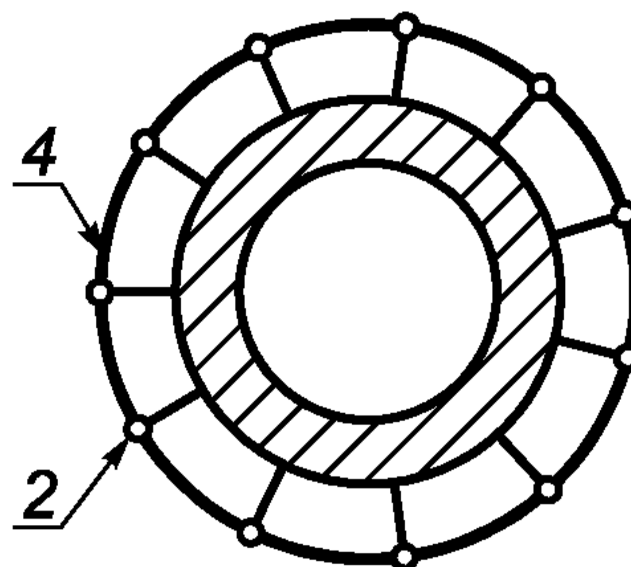
б) Анкерное устройство, устанавливаемое, например, на трубе
